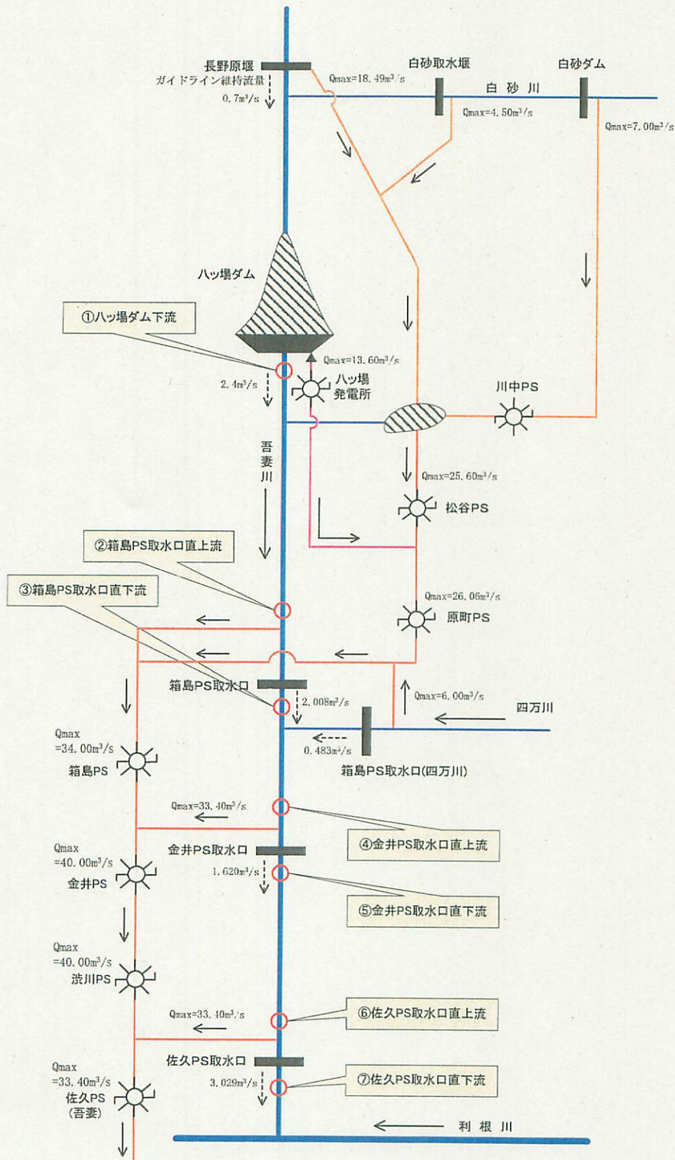
図-4 ハッ場ダム下流における発電取水系統
