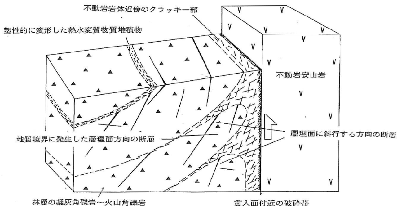
第5図 資料（2）による白岩沢周辺斜面の構造地質の模式図
