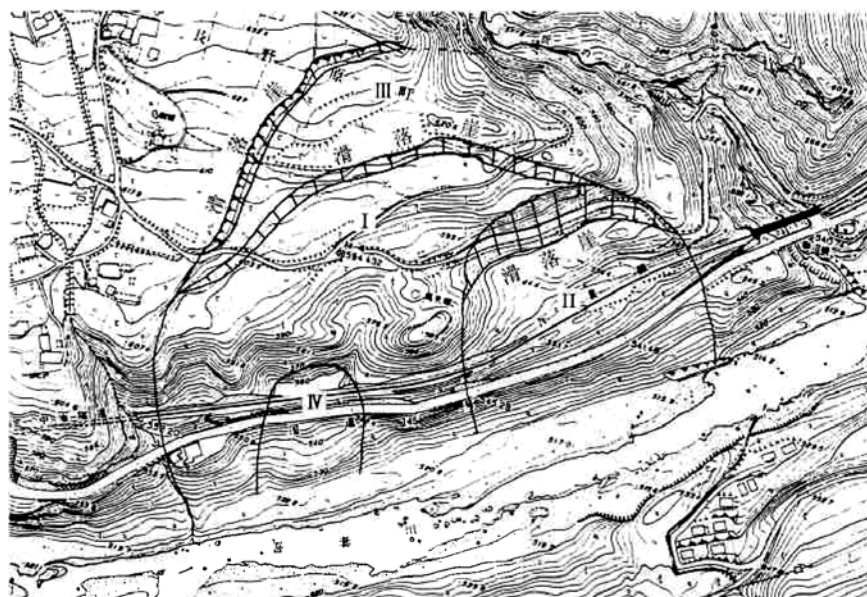
第4図 過去の地すべり記録に基づく林地地区地すべり平面図（長野原町教育委員会「長野原の自然」より）
