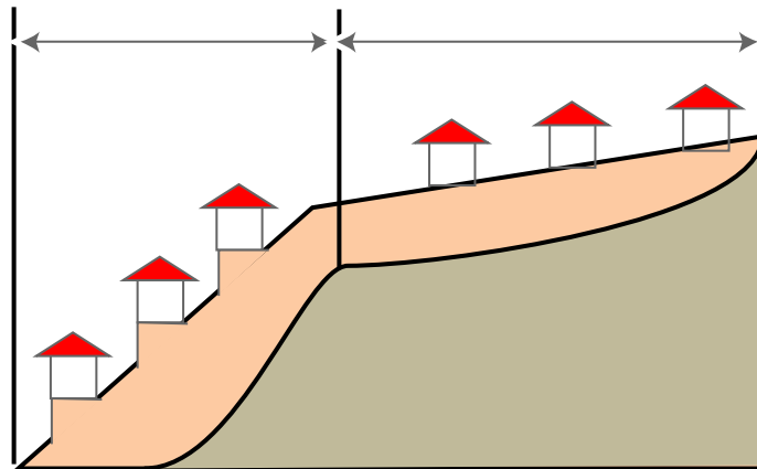
図参 5.1-⑥ 地形変換点における大規模盛土造成地の区分（縦断面）
