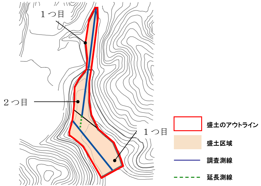
図参 5.1-⑤ 地形変換点における大規模盛土造成地の区分
