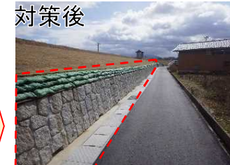
堤防強化対策の事例 （阿賀野川水系阿賀野川）
