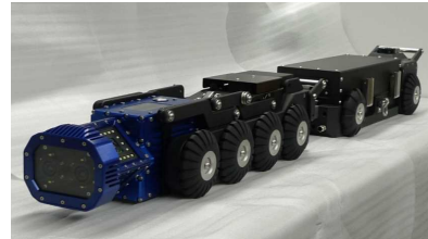
下水道管路の欠陥を画像認識技術により自動検出するロボット
