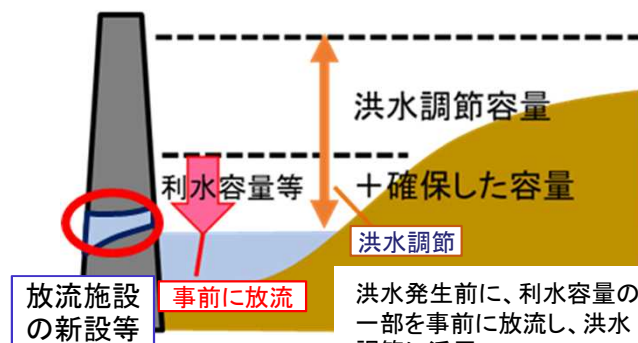
事前放流のイメージ
