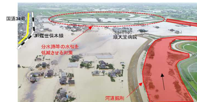
河道掘削の実施
